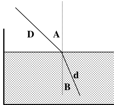
Figura 1 - Quando a luz passa de um meio menos refringente (como o ar) para outro mais refringente (como a água) ela se desvia, obedecendo à lei de Snell-Descartes. Maupertuis procurou explicar a refração através do princípio de ação mínima.
