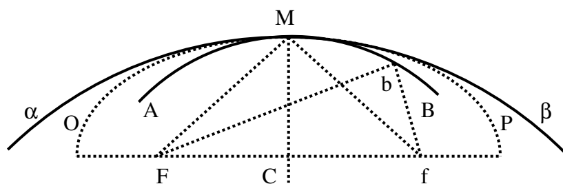
Figura 2 - Esquema geométrico publicado por Patrick d'Arcy, para mostrar que na reflexão da luz por um espelho côncavo o percurso seguido pela luz pode ser o caminho máximo, em vez de mínimo.
