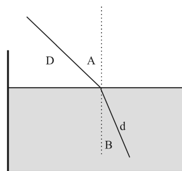
Figura 1 - Quando a luz passa de um meio menos refringente (como o ar) para outro mais refringente (como a água) ela se desvia, obedecendo a lei de Snell-Descartes. Maupertuis procurou explicar a refração através do princípio de ação mínima.
