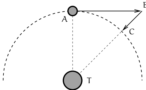
Figura 4 Esquema do movimento da Lua em torno da Terra, indicando o movimento que ela teria se não fosse empurrada ou puxada na direção da Terra (AB) e a sua “queda” da tangente para a trajetória circular (BC), em direção à Terra (T).
